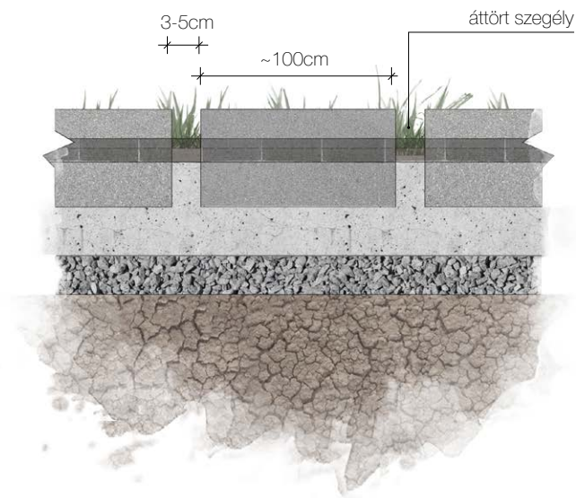
12 ábra: Áttört szegély metszet/oldalnézet
