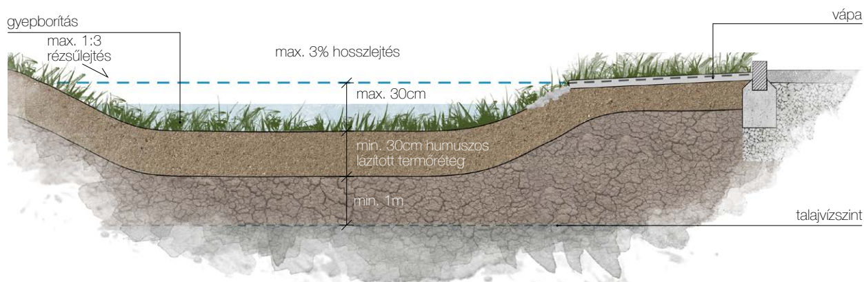
20. ábra: Szikkasztóárak metszet
