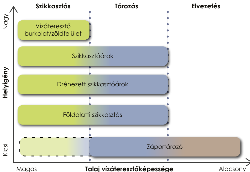
10. ábra Eszközök alkalmazhatósága a rendelkezésre álló hely és a talaj vízáteresztő képességének függvényében (H. Dreiseitl, W. Geigner, 2012)
