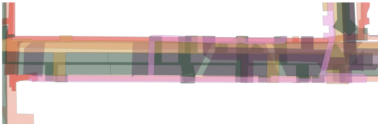
47. ábra: A közmujszáló védőtávolsága összegezve, faültetés csak kompromisszummal volt lehetséges
