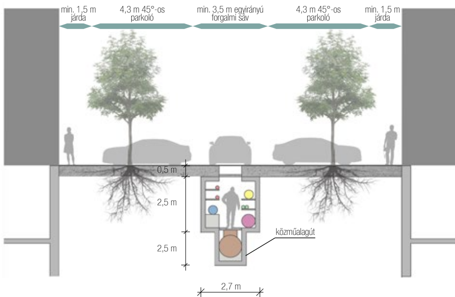
18. ábra: Egyirányú utca mintakeresztmetszévénye, kétoldali 45°-os parkolóval közmuívekkel, ideális megoldás
