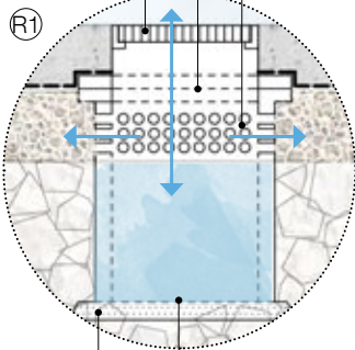
33. ábra: Stockholmi fahely modell a 2,25 m 2 -es fahely szerint adaptálva légáteresztő teherhordó réteg zúzottkő (32-63 mm) esővíz szivargó, levegőztető műtárgy "stockholmi" szegélyelem R1 R2 0,4-0,8 m 1,5 m talajilazítás 0,2 m vastagságban faveremrács termőtalaj burkolat geotextília 0,2 m 0,8 m zúzottkő réteg (100-150 mm), mely közé termőtalaj kerül bemosásra légáteresztő teherhordó réteg zúzottkő (32-63 mm)
